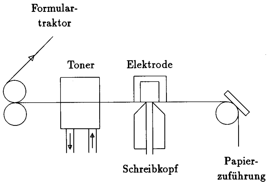
Prinzip des elektrostatischen Plotters
