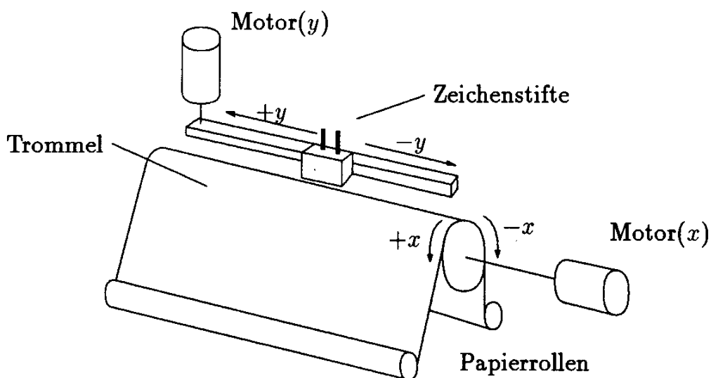
Prinzip des Trommelplotters
